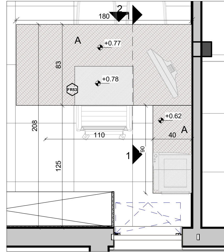
1 שולחן חדר רופא 1 : 20
