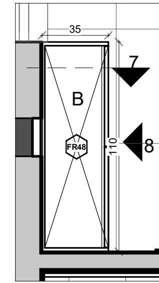
1 ארון חדר הדרכה 1 : 20
