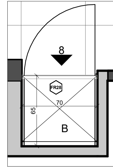
1 ארון - חדר טיפולים 1 : 20
