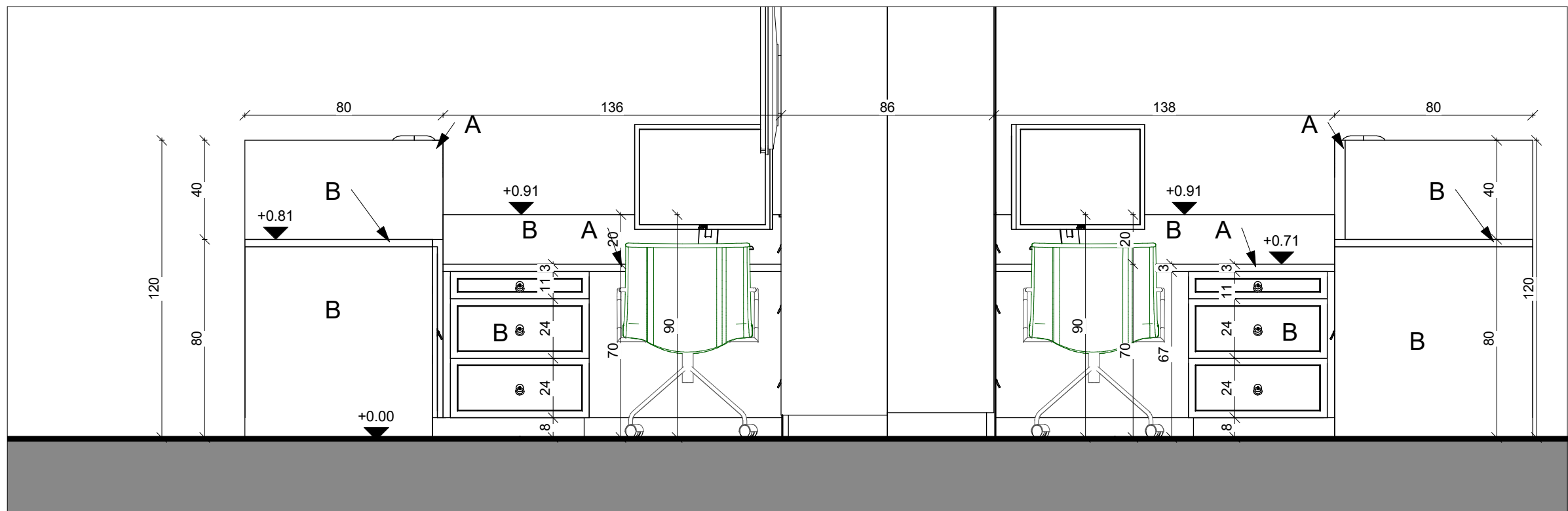
עמדת אחיות 1 - פרישה 2 1 : 20
