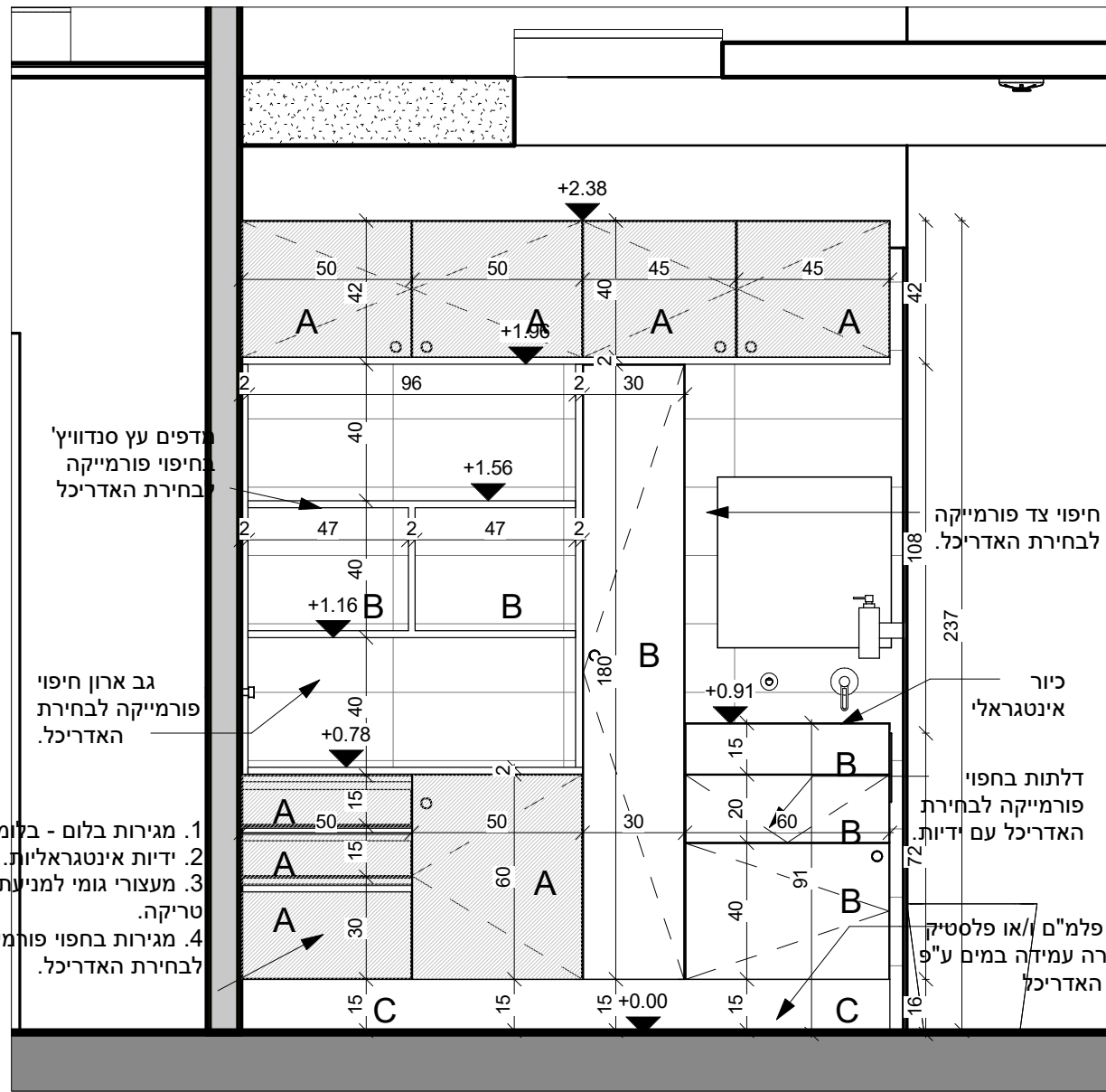
פרישה 2 - 1:20 2
