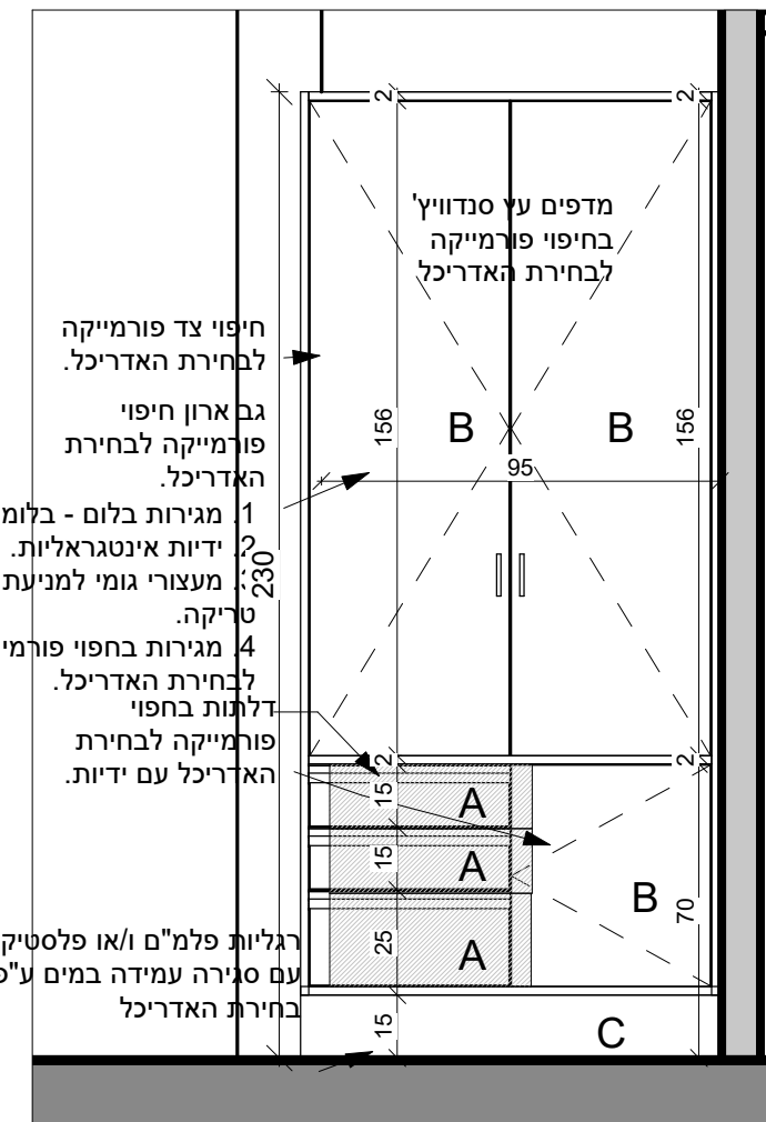
3 פרישה 6 1 : 20
