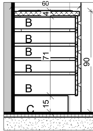
4 חתך 6-6 1 : 20
