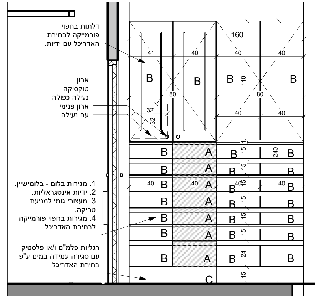
פרישה-9 2 1:20
