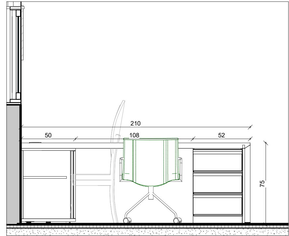
פרישה-8 1 : 20 ②
