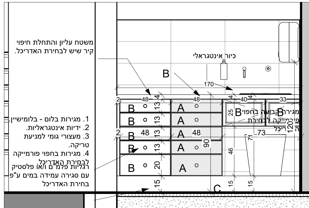
2 פרישה 11 1 : 20
