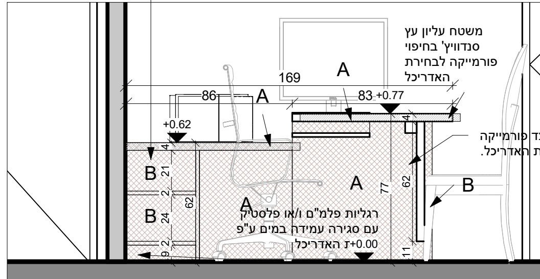
חתך 2-2 2 1 : 20
