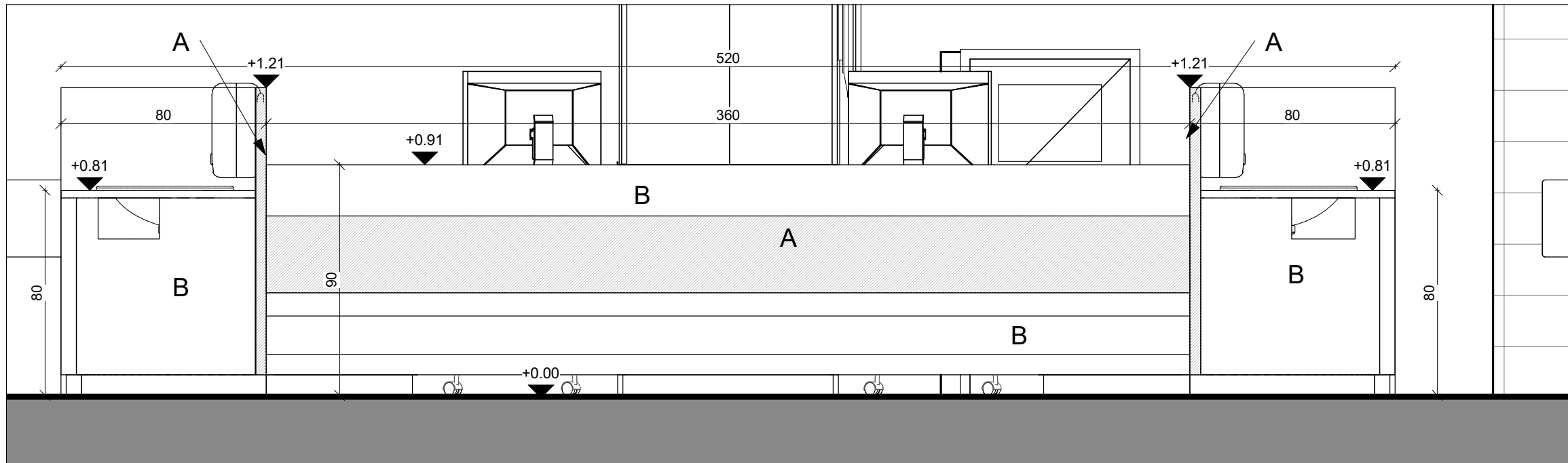
עמדת אחיות 1 - פרישה 1 1 : 20
