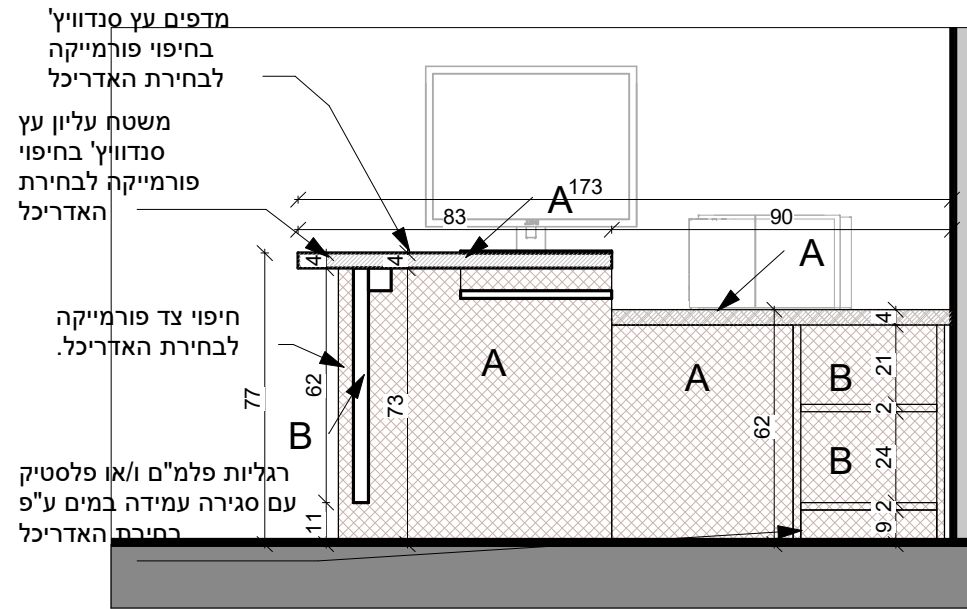
3 חתך 3-3 1:20
