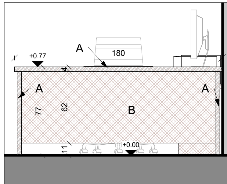
פרישה-4 4 1 : 20
