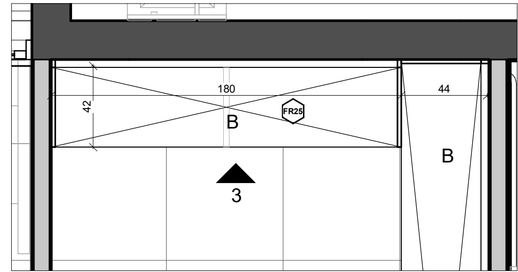
1 ארון מחסן 1:20
