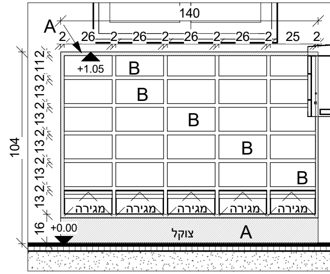
2 פרישה--2 1 : 20
