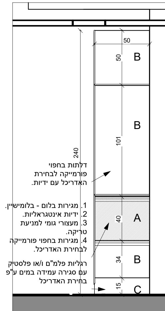
ארון עמדת אחיות 1 3
