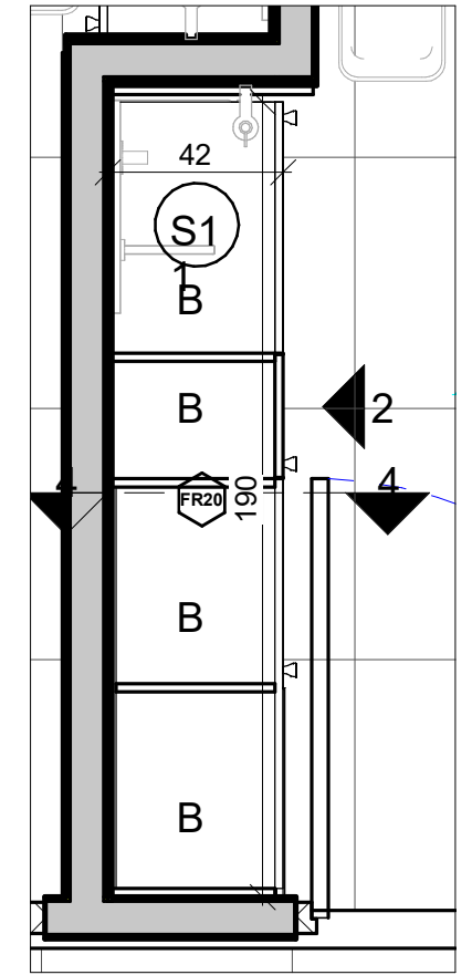
ארון חדר טיפולים 2 1:20 1
