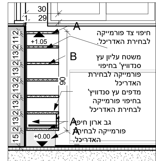
4 חתך 5-5 1 : 20
