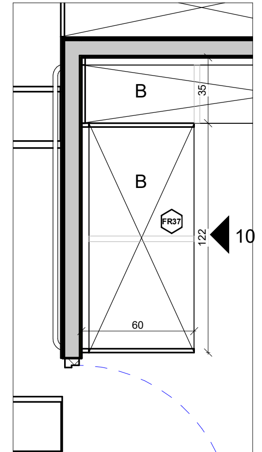
1 ארון מחסן רפואי 1 1:20
