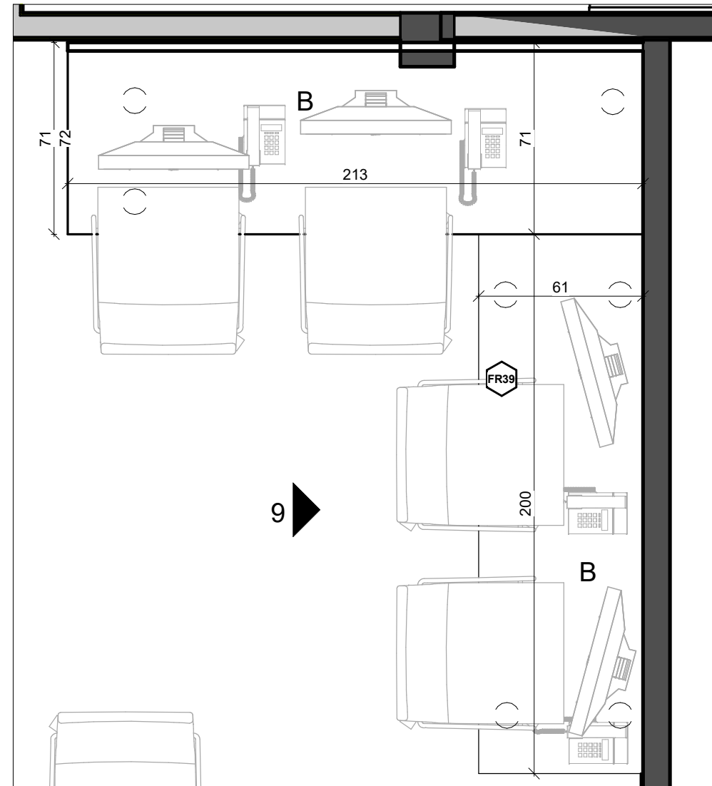
עמדת אחיות 1 1 : 20
