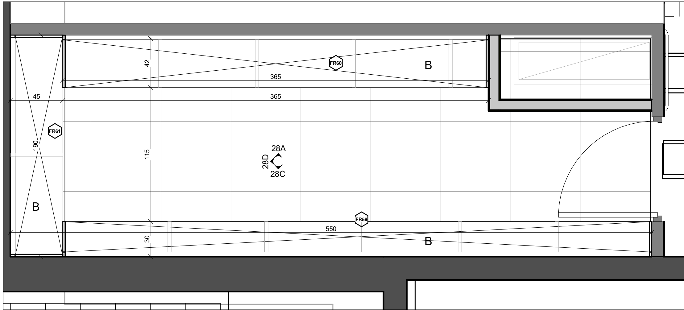
1 ארון מחסן מש' 1 1 : 20
