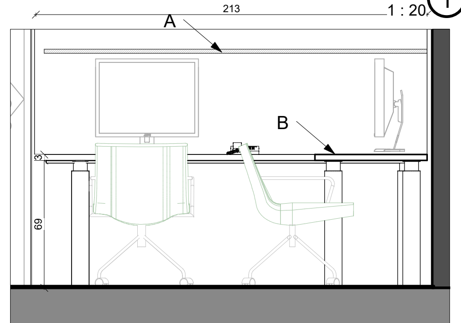
חתך 5-5 (4) 1 : 20
