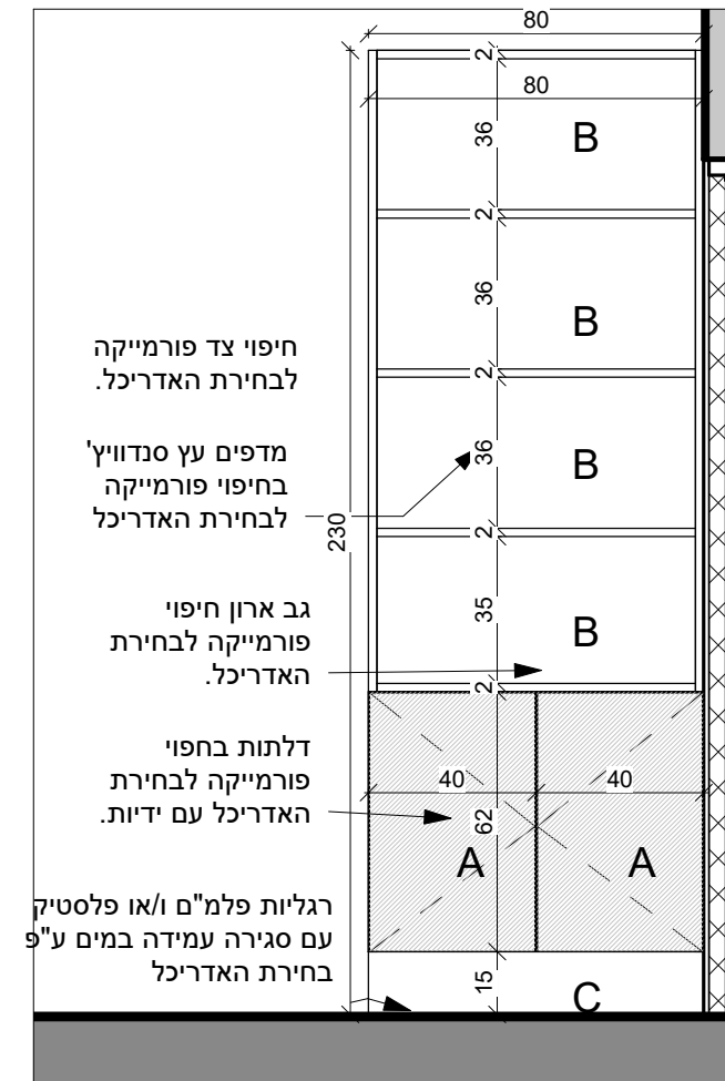
פרישה 14 1 : 20
