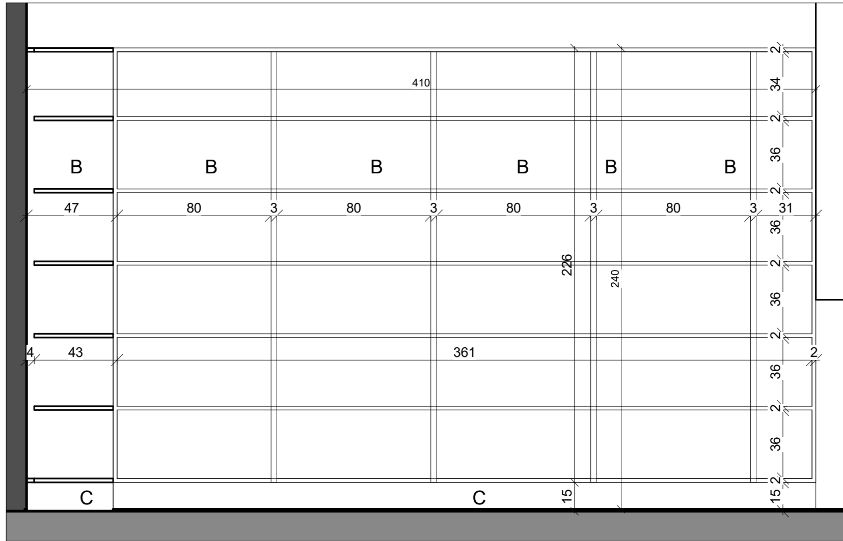
28.A 2 1:20
