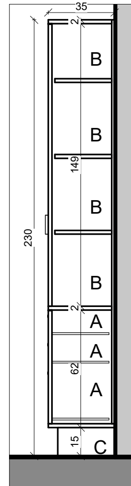
4 חתך 7-7 1 : 20
