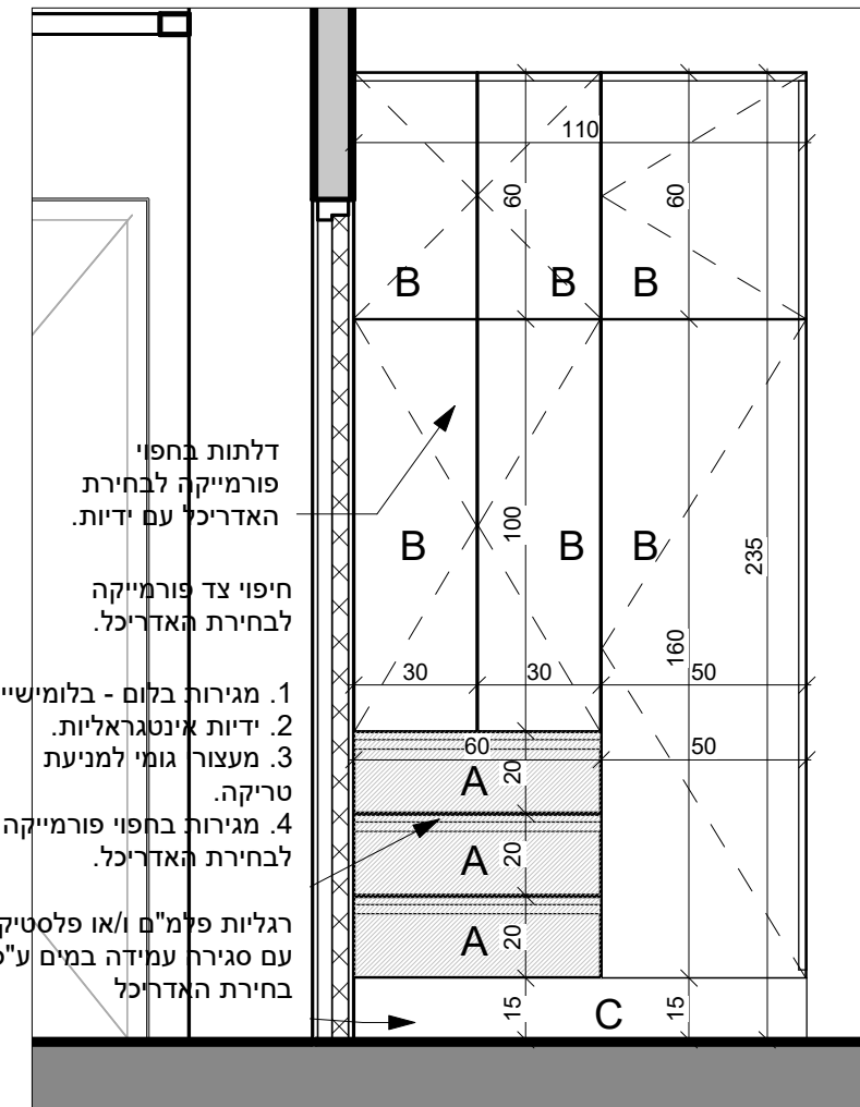
2 פרישה 5 1:20
