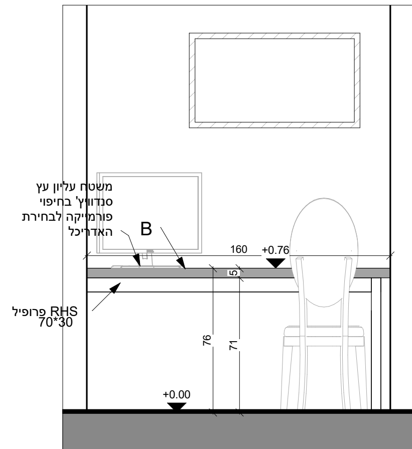
פרישה--3 1 : 20
