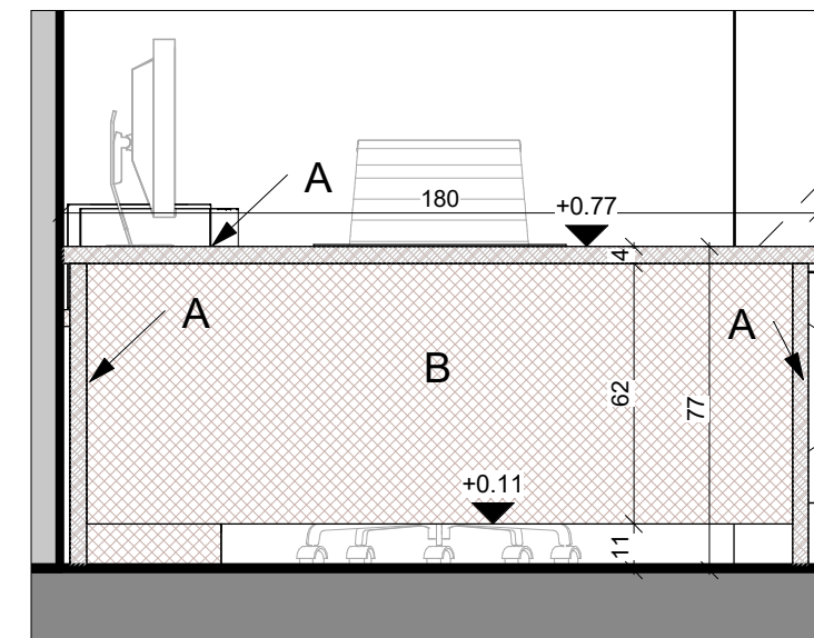
4 פרישה 4 1:20
