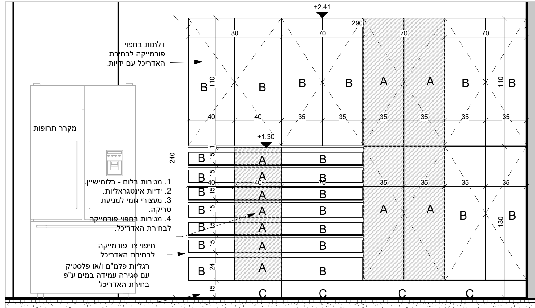
ארון תרופות מחקרים - פרישה 1 1 : 20
