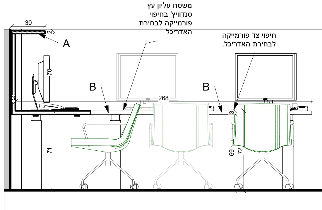
פרישה 9- 2 1 : 20
