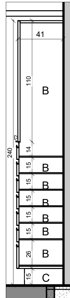
חתך 8-8 4 1:20
