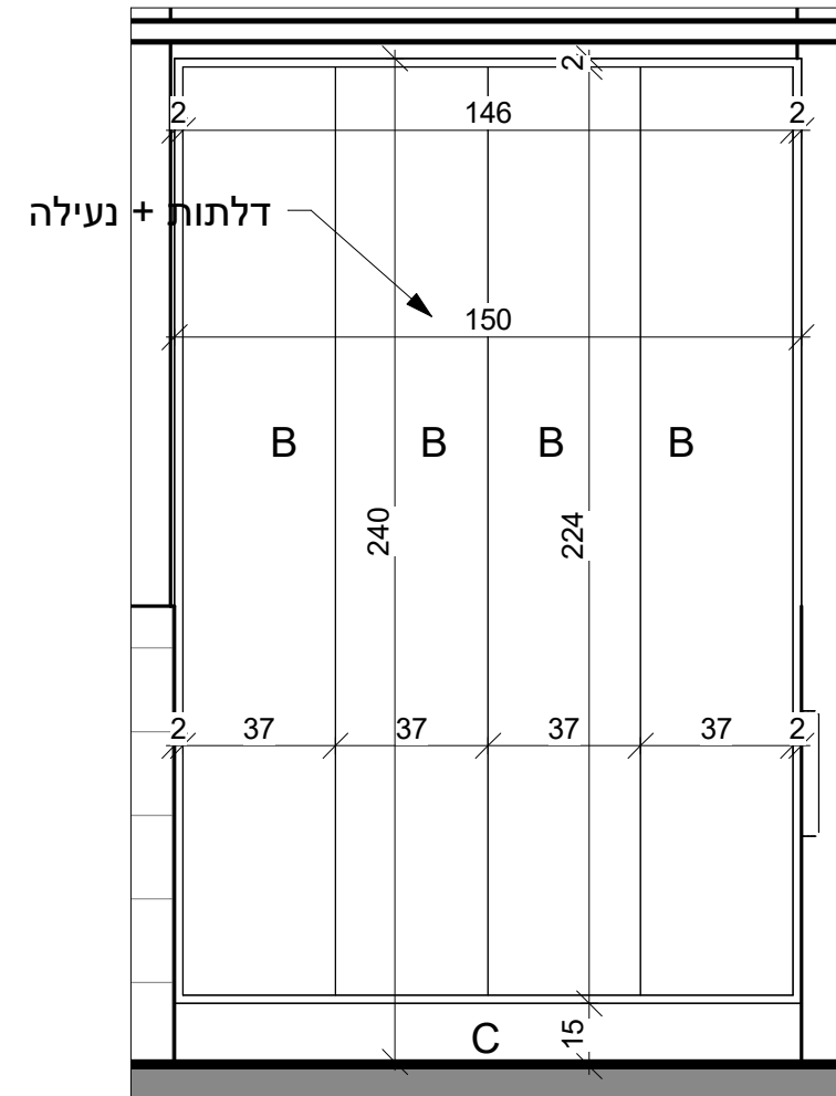
2 פרישה-2 1 : 20
