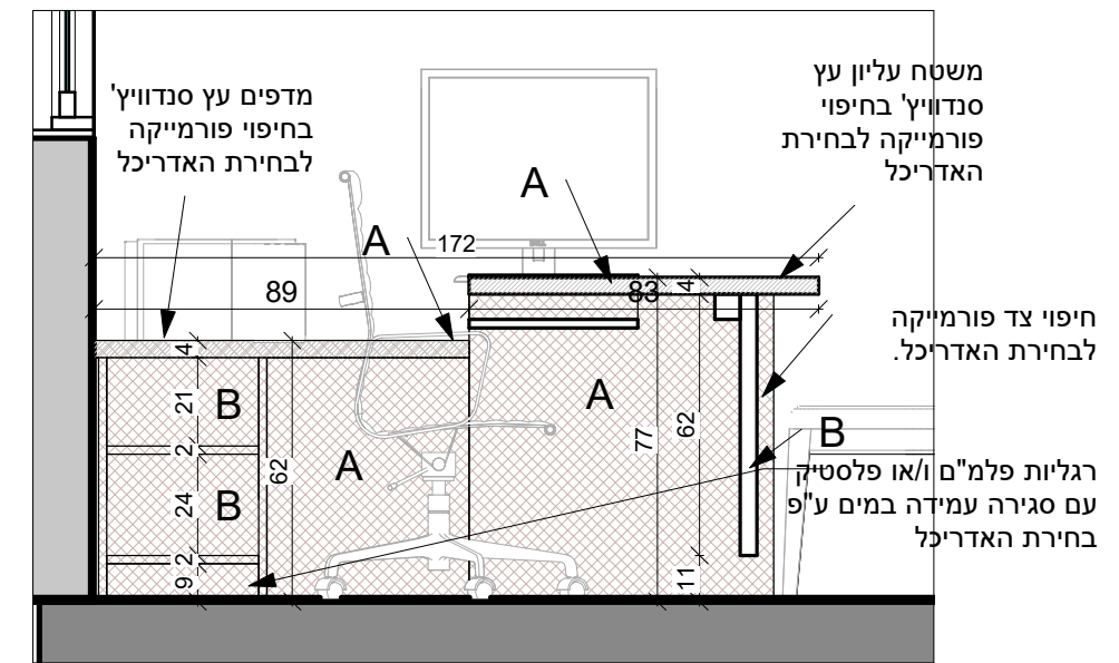
חתך 6-6-4 1:20
