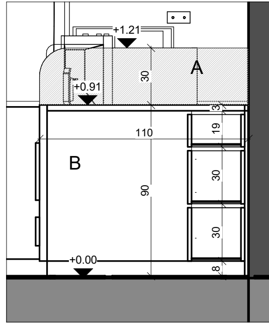
עמדת אחיות 1 - חתך 2 5 1 : 20
