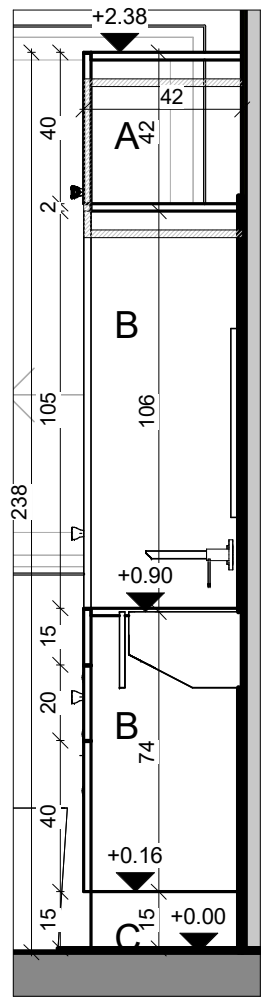
חתך 4-4 1 : 20
