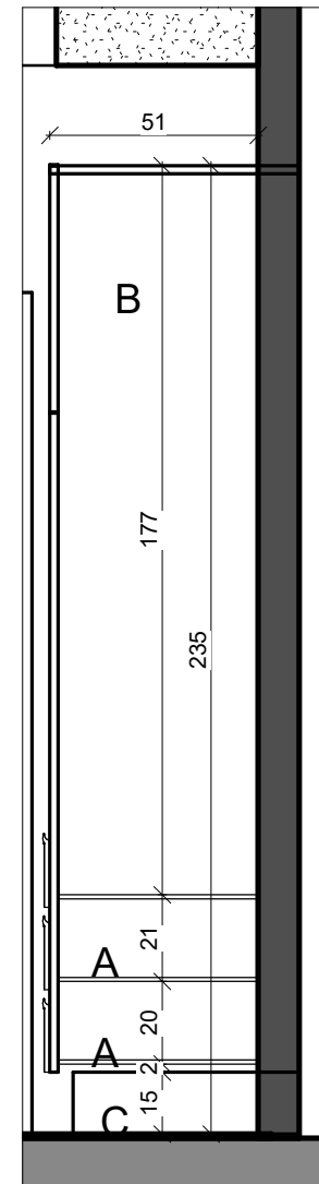
4 חתך 6-6 1:20
