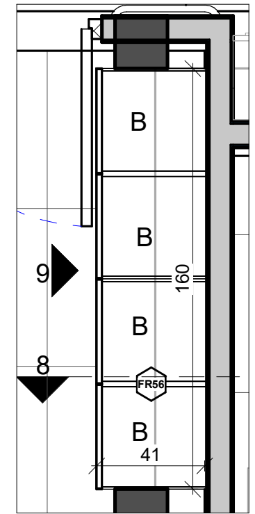
ארון תרופות 1 1:20
