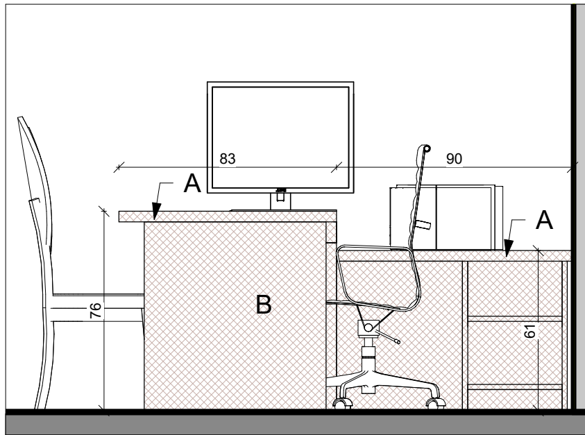
פרישה 1 1 : 20 5
