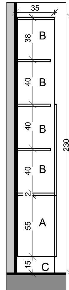
חתך-5-5 1 : 20
