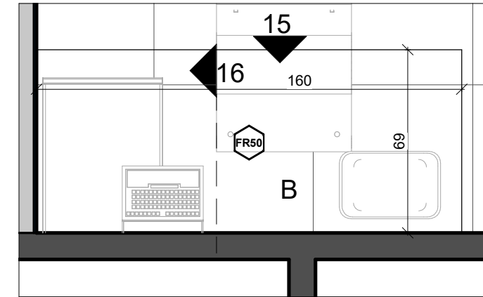
שולחן עבודה רופא תורך 2 1 1 : 20
