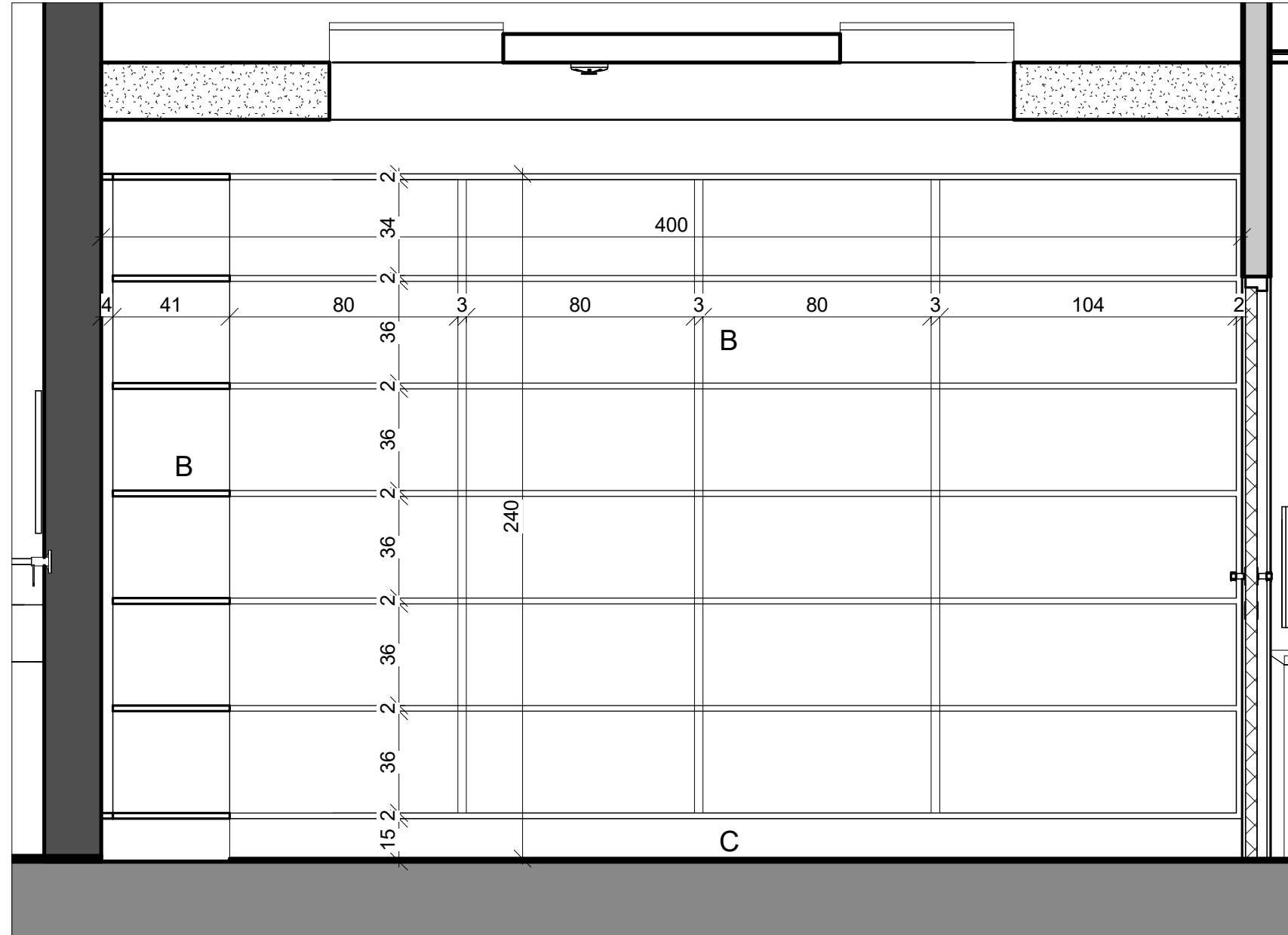
פרישה 2 1 : 20
