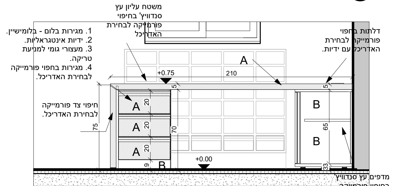
4 פרישה 7 1:20
