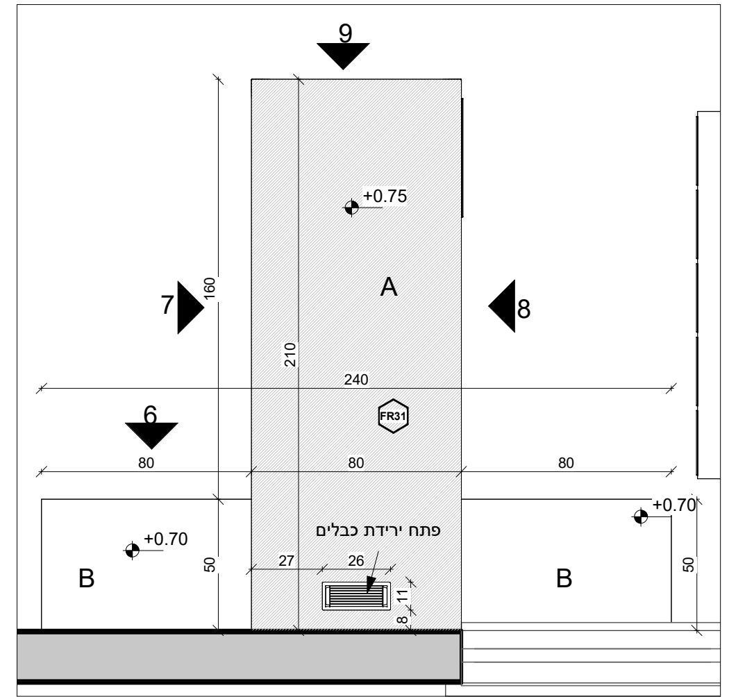
1 שולחן עבודה מחקרים 1:20
