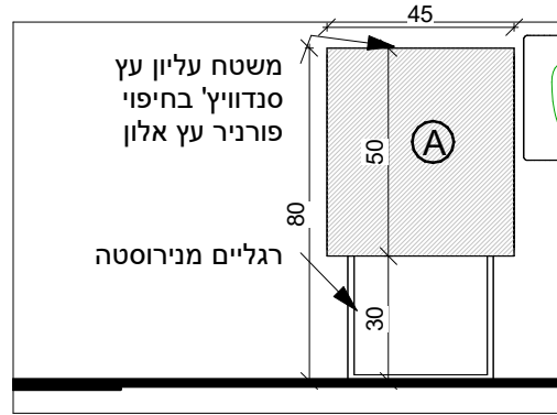
4 ארון המתנה - פרישה 3 1 : 20
