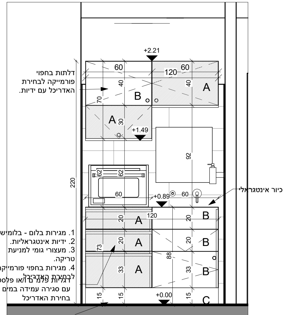
2 פרישה 2 1 : 20
