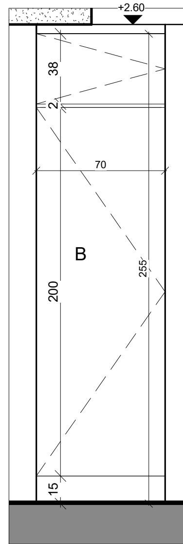
3 פרישה 8 1 : 20
