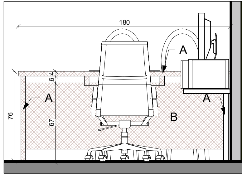
פרישה 3 - 5 1 : 20
