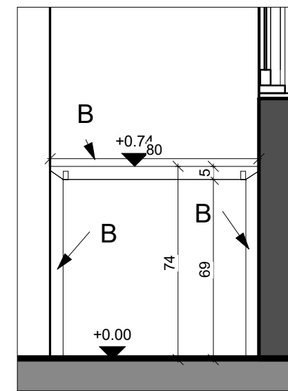
3 פרישה-3 1 : 20
