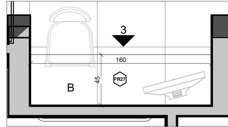
שולחן חדר טיפולים 1 1 : 20
