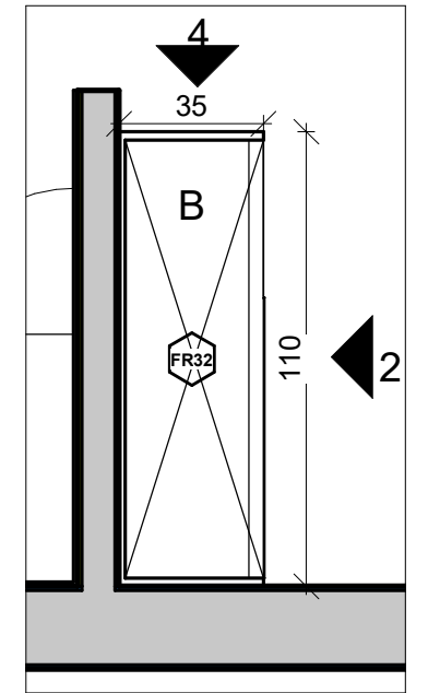
1 ארון מחקרים 1:20
