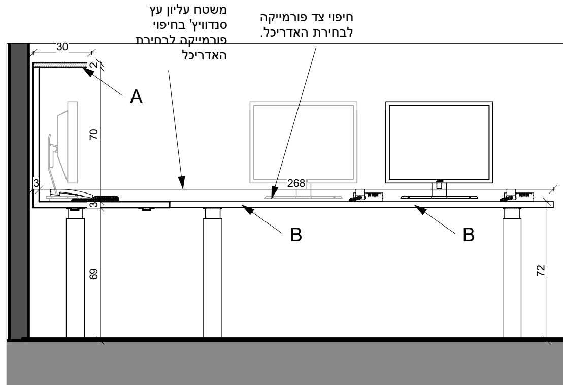
חתך 5-5 (2) 1 : 20
