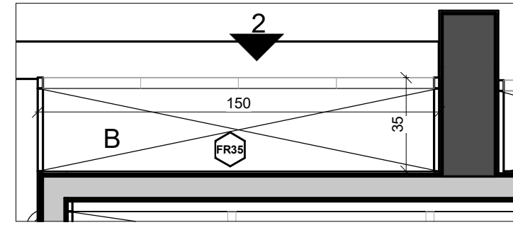
1 ארון מסדרון 1 : 20
