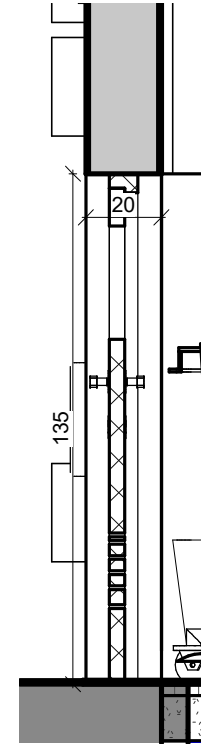
2 חתך 6-6 1 : 20
