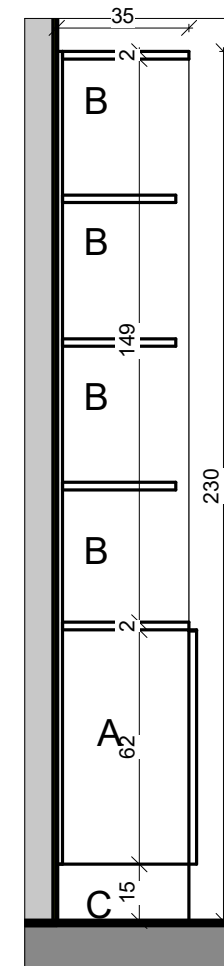
חתך 15-15 1 : 20
