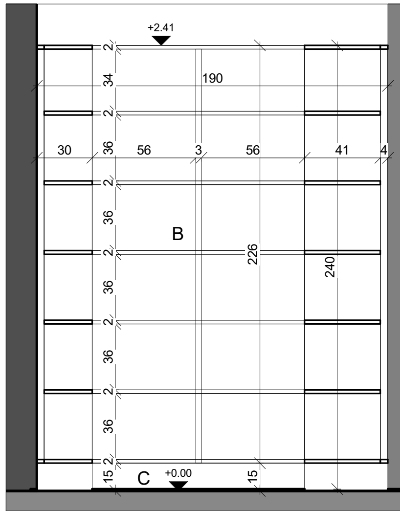
28.D 1 : 20 (2)
