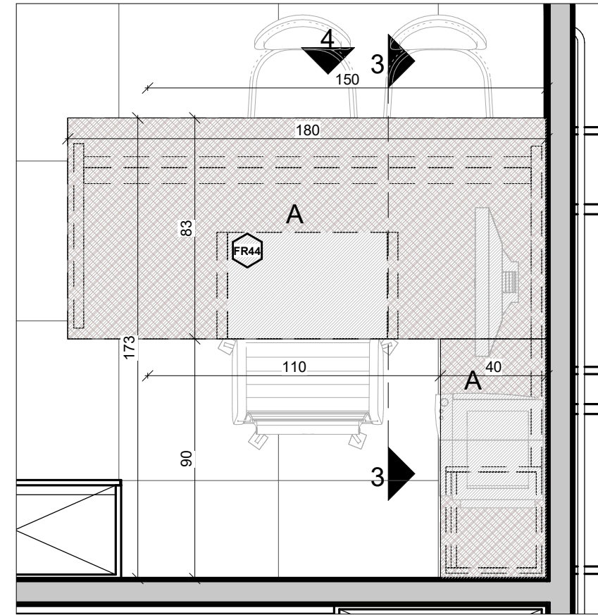
1 שולחן חדר הדרכה 1:20
