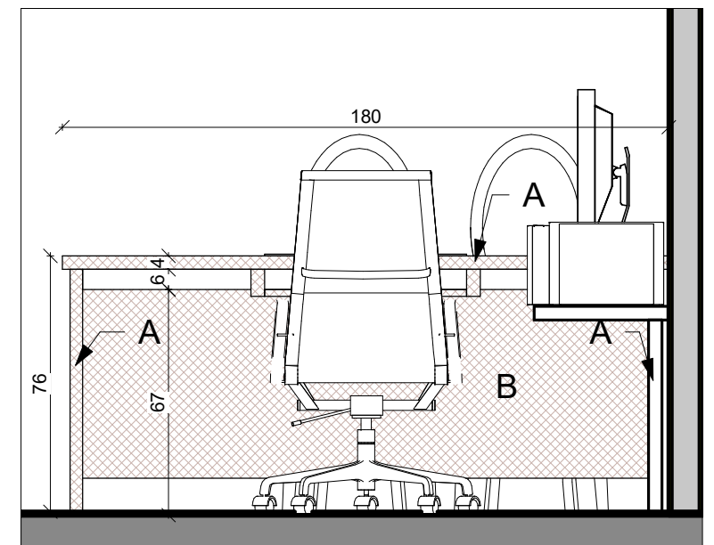
פרישה 3 1 : 20 6
