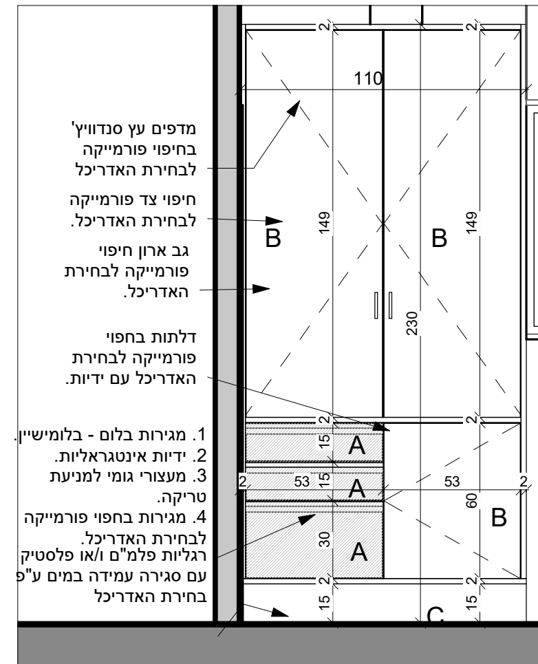
2 פרישה 8-- 1 : 20
