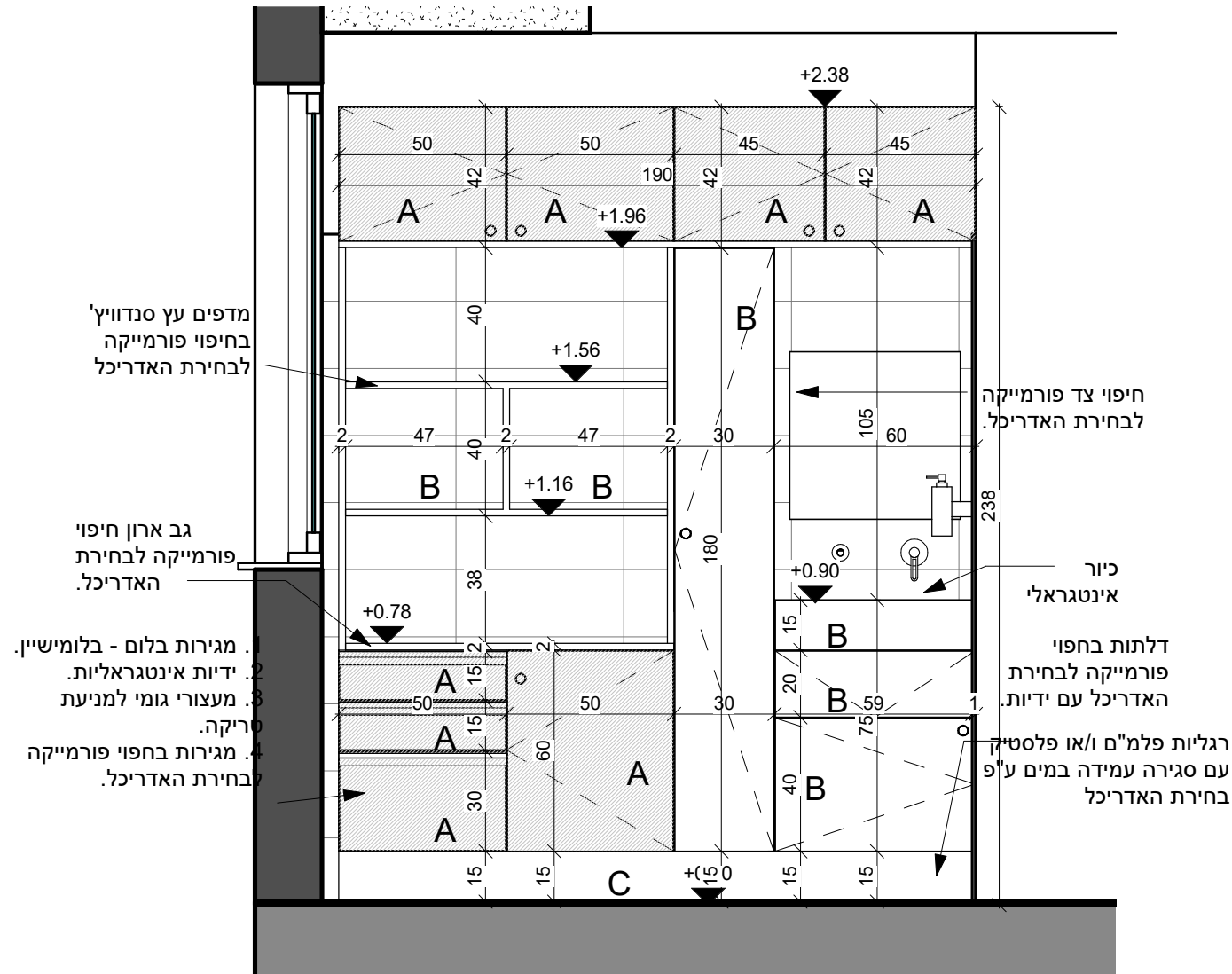
פרישה-2 1 : 20
