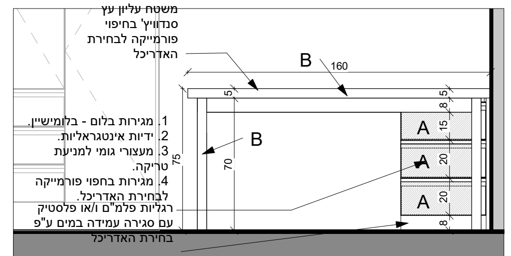
פרישה 15 2 1 : 20
