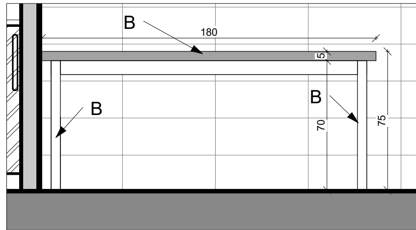
PD משטח עבודה 3 1 : 20
