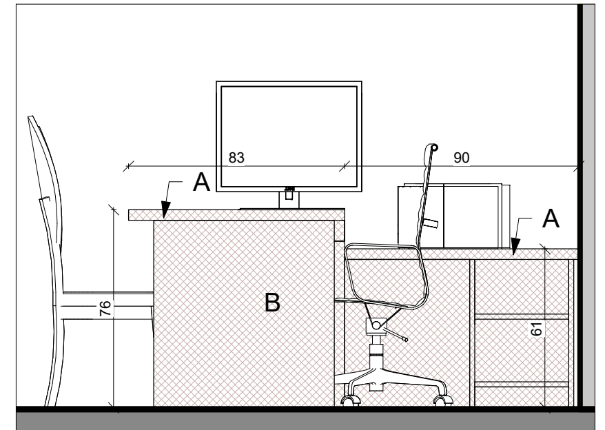
פרישה-1 3 1 : 20
