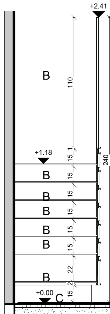
ארון תרופות מחקרים - חתך 1 : 20
