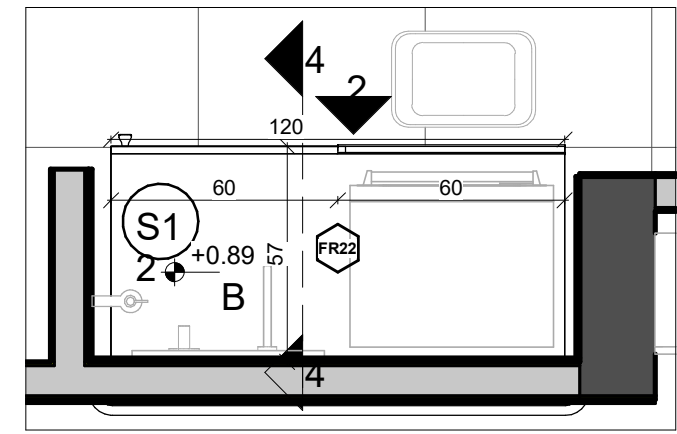
1 ארון תנור 1 : 20
