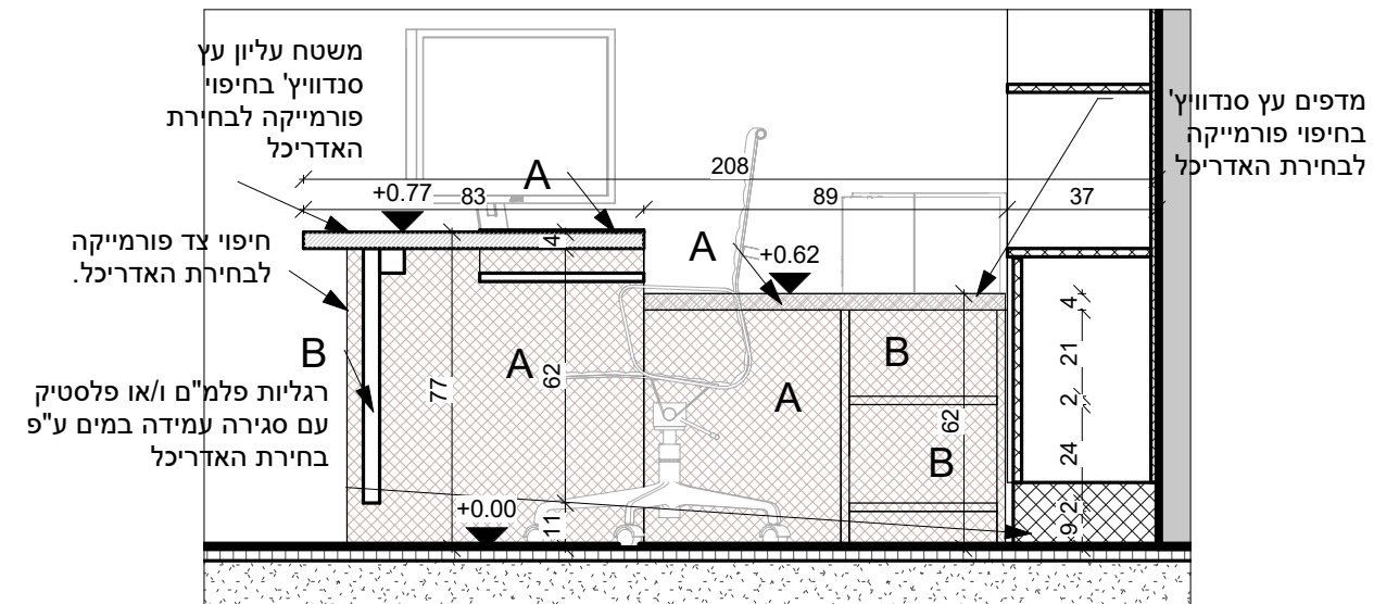
4 חתר..1-1 1 : 20
