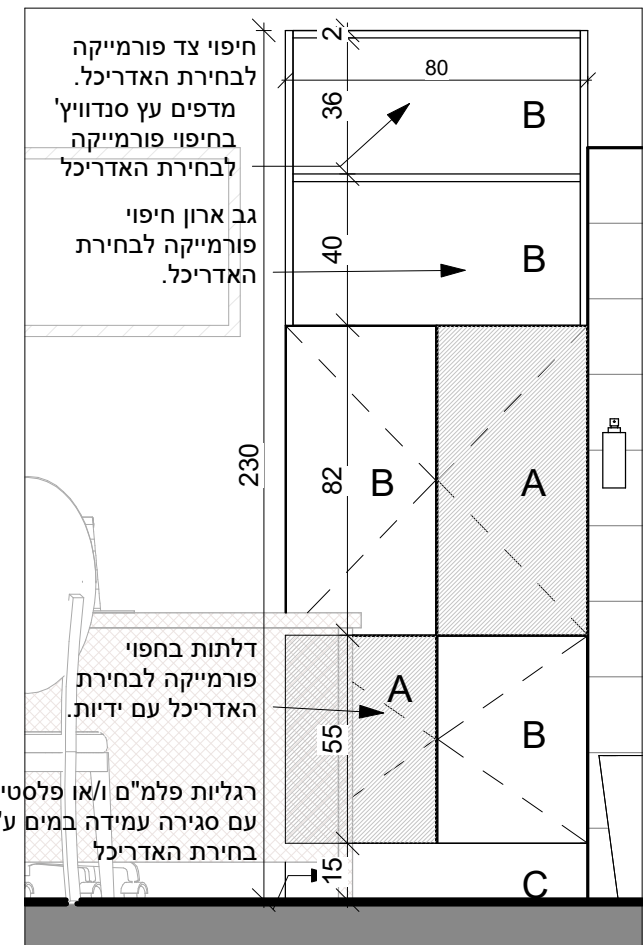
פרישה 9 1 : 20
