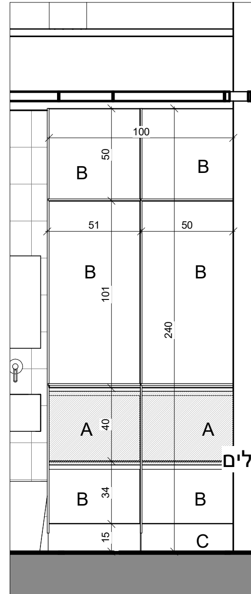
2 פרישה 1 : 20
