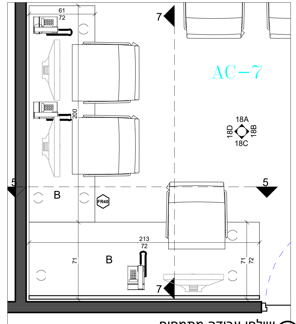
שולחן עבודה מתמחים (1) 1 : 20
