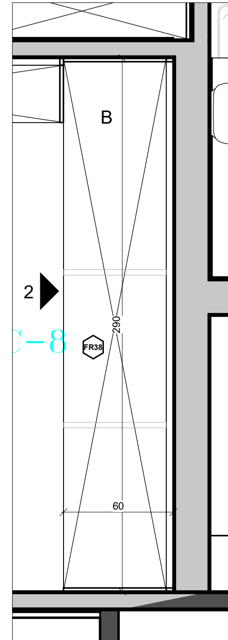
1 ארון מחסן רפואי 3 1:20
