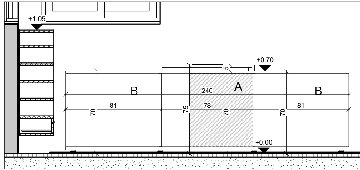
2 פרישה 6 1:20
