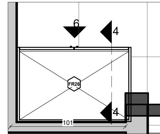
1 ארון-חדר טיפולים 1 : 20
