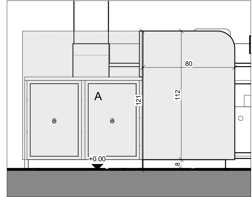
עמדת אחיות 1 - חתך 1 3 1 : 20
