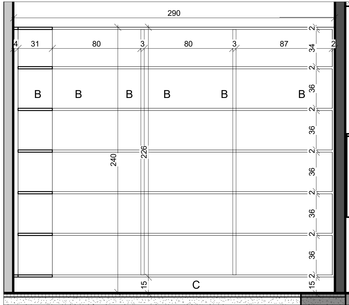
2 פרישה*2 1:20
