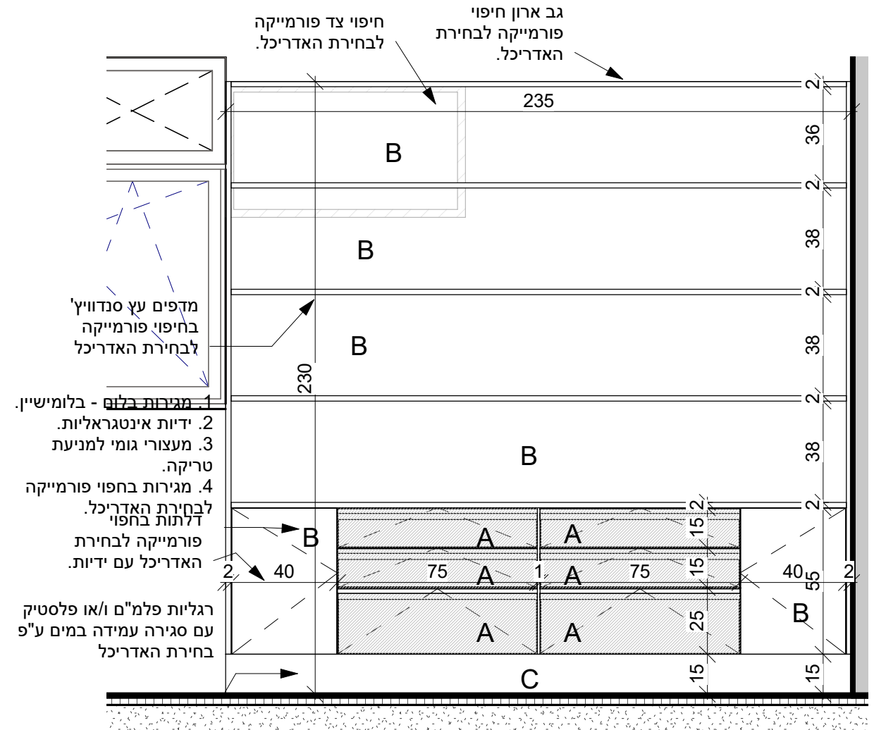
2 פרישה 7 1 : 20
