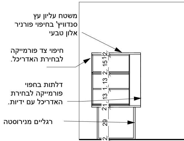
5 חתך ארון ב 1 : 20
