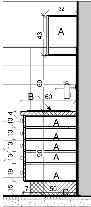
3.3 חתך 1:20
