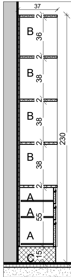
4 חתך 3-3 1 : 20
