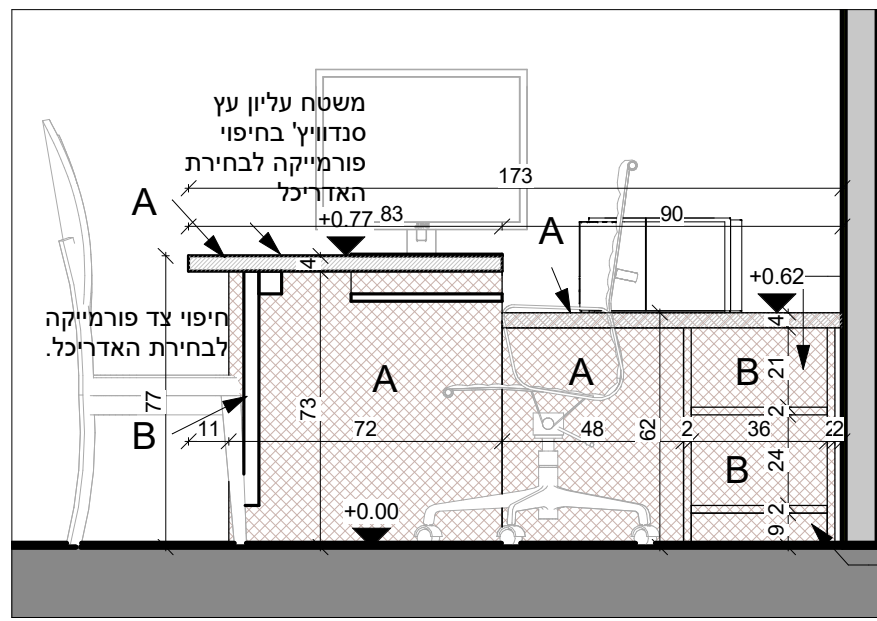
חתך 2-2 1 : 20 2
