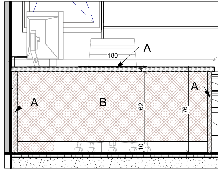
2 פרישה-1 1 : 20
