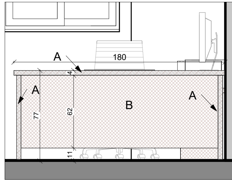
פרישה-7-2 1:20
