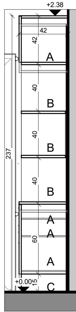
חתך 4-4 1:20 4
