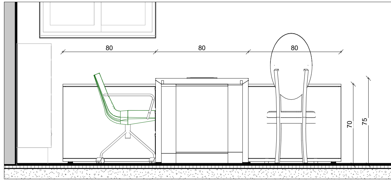
פרישה 9 1 : 20 ①
