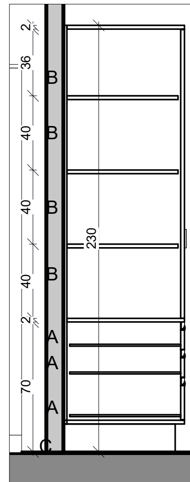
4 חתך-4-4 1 : 20
