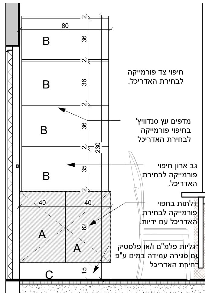
2 חתך 1-1 1 : 20
