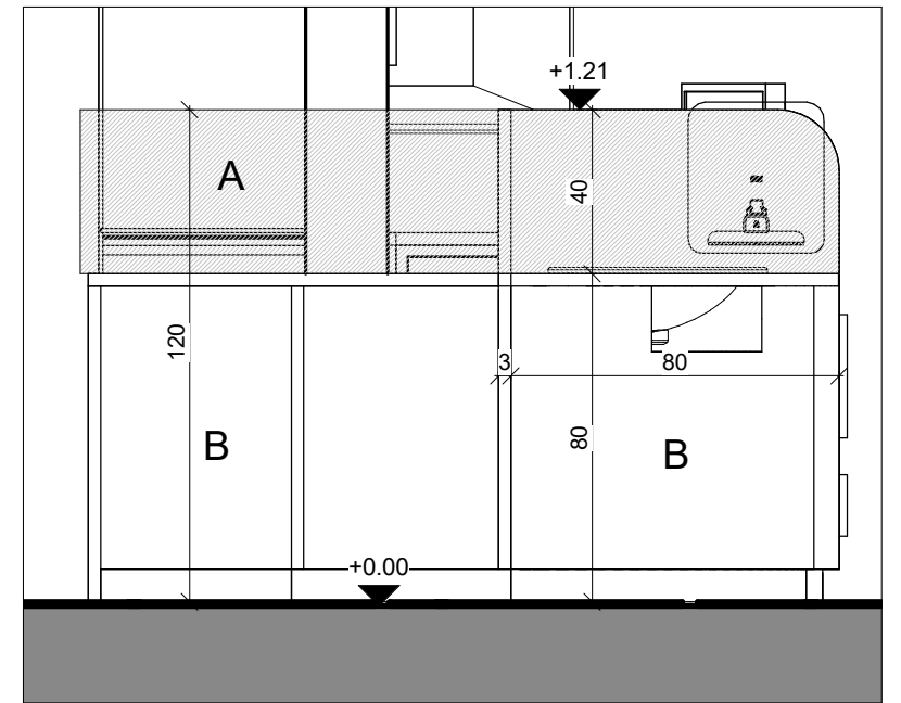
עמדת אחיות 1 - חתך 3 4 1 : 20
