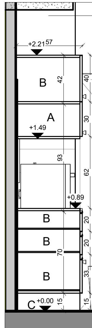
4 חתך 4-4 1 : 20
