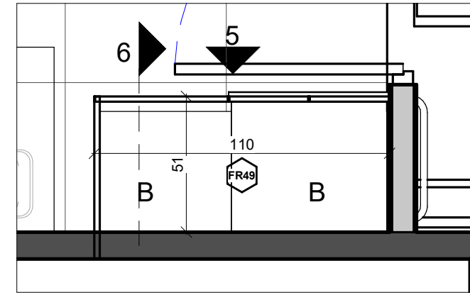
1 ארון חדר רופא תורן 1:20
