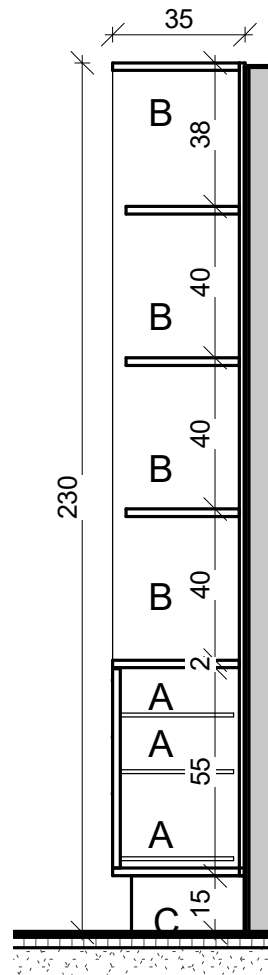
4-4 חתך 1:20
