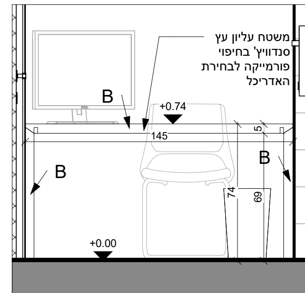
3 פרישה 5 1 : 20
