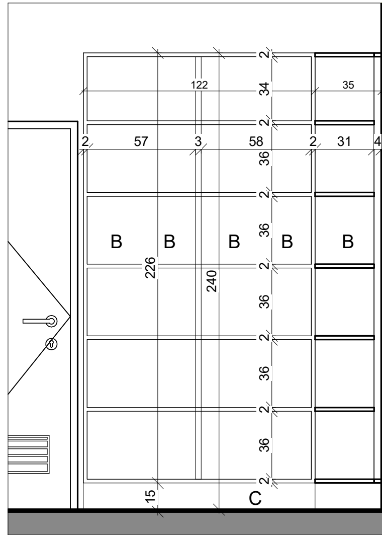
2 פרישה 10 1:20
