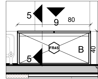
ארון חדר הדרכה 2 1 : 20
