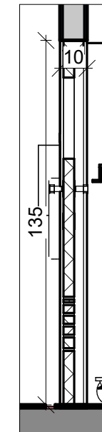
חתך-1-1 1 1 : 20
