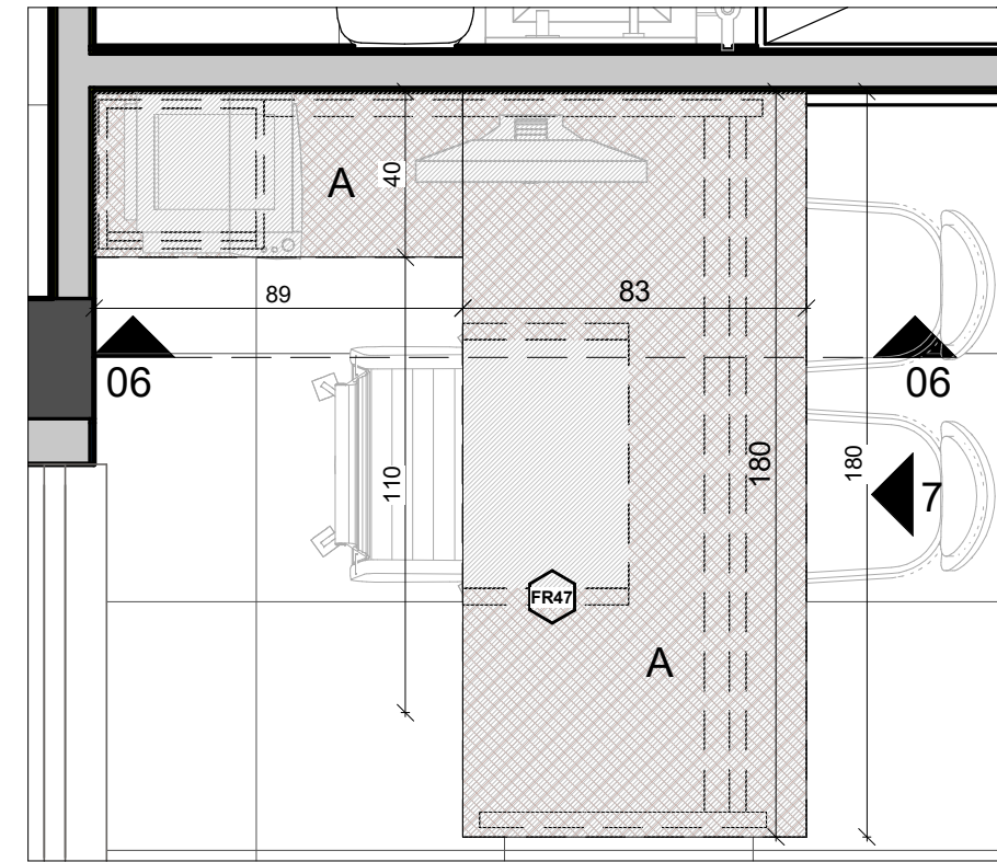
שולחן עבודה - חדר הדרכה 1 1:20
