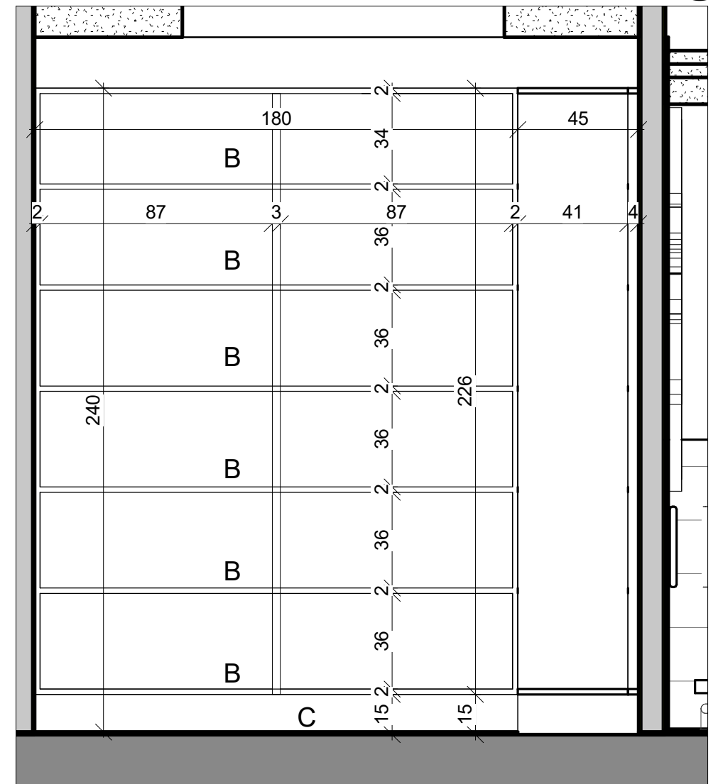
3 פרישה 3 1:20
