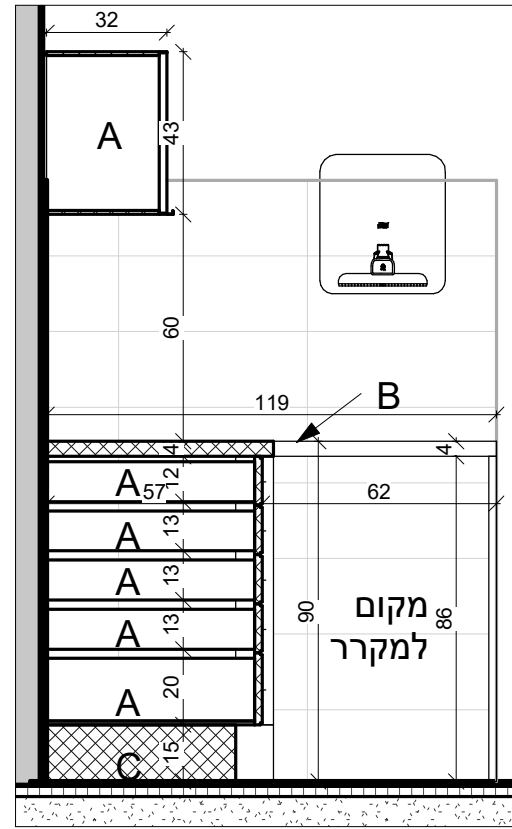
5-5 חתך 1:20
