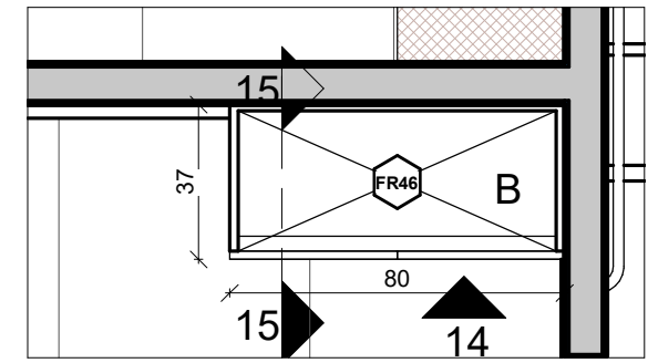
ארון חדר הדרכה 1 1 : 20
