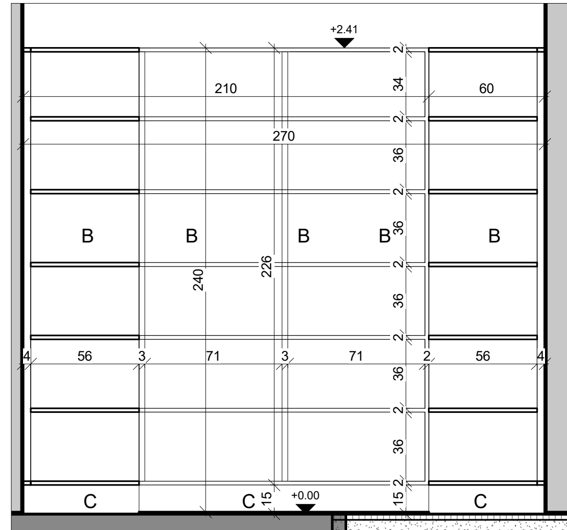
1 ארון מחסן רפואי 1:20
