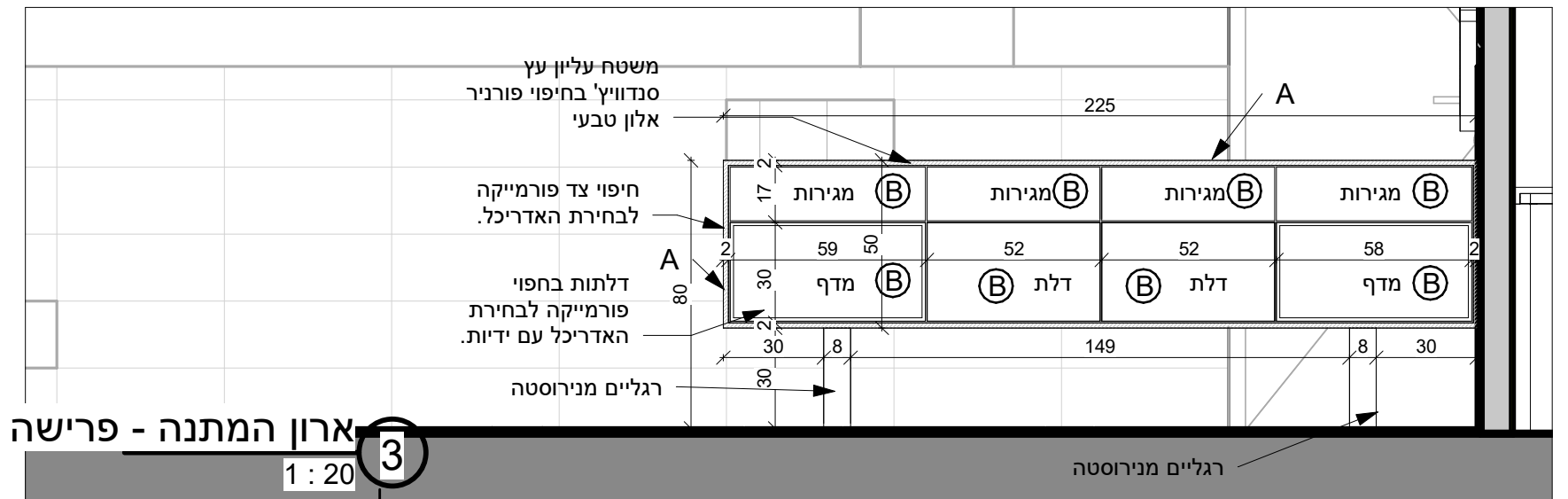
ארון תצוגה באולם המתנה
