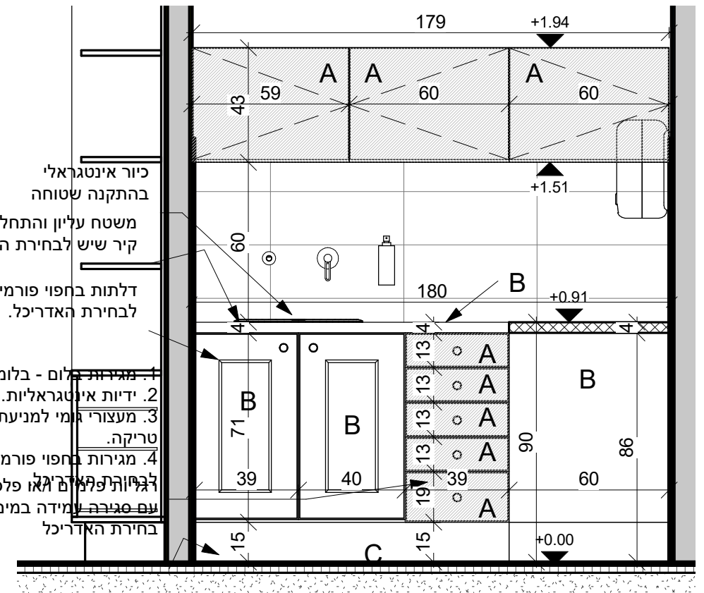
2 פרישה 1:20
