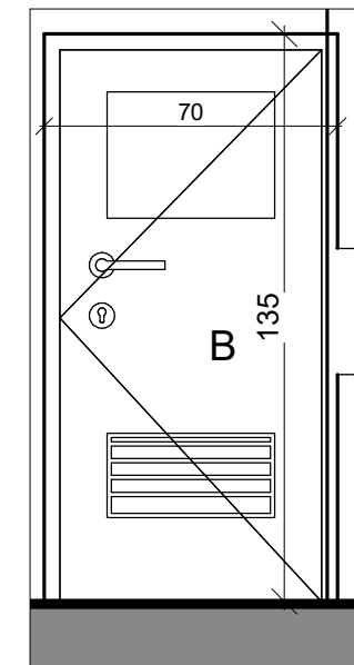
פרישה 1 4 1 : 20
